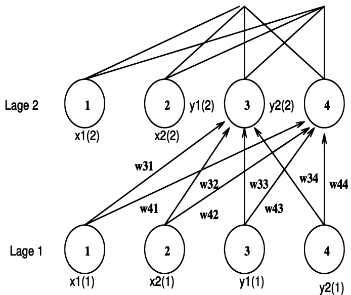
Abbildung 1.1: Links ist ein zyklisches Netz dargestellt, welches zu einem azyklischen Netz entfaltet wird, welches rechts dargestellt ist. Es werden p Schritte zurueckpropagiert, wodurch man p+1 Lagen im azyklischen Netz erhalt. Die Knoten 1 und 2 sind Eingabeknoten und die Knoten 3 und 4 sind rekurrent. In der Lage p+1 ist die Aktivierung der Eingabeknoten beliebig, da diese Aktivierung nicht verwendet wird.
